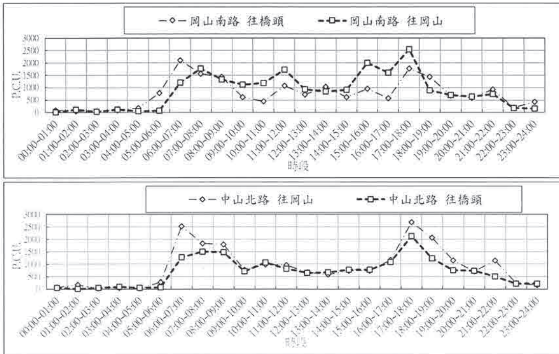
圖2.6-1 各測站交通流量逐時變化圖
