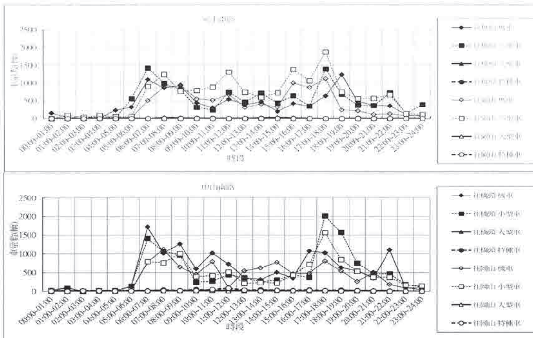
圖2.6-2 各測站車種逐時變化圖
