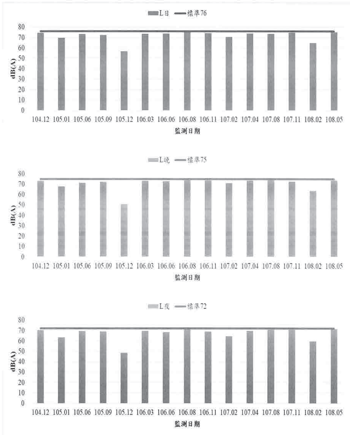
圖2.2-2 橋頭社區醫院噪音監測結果
