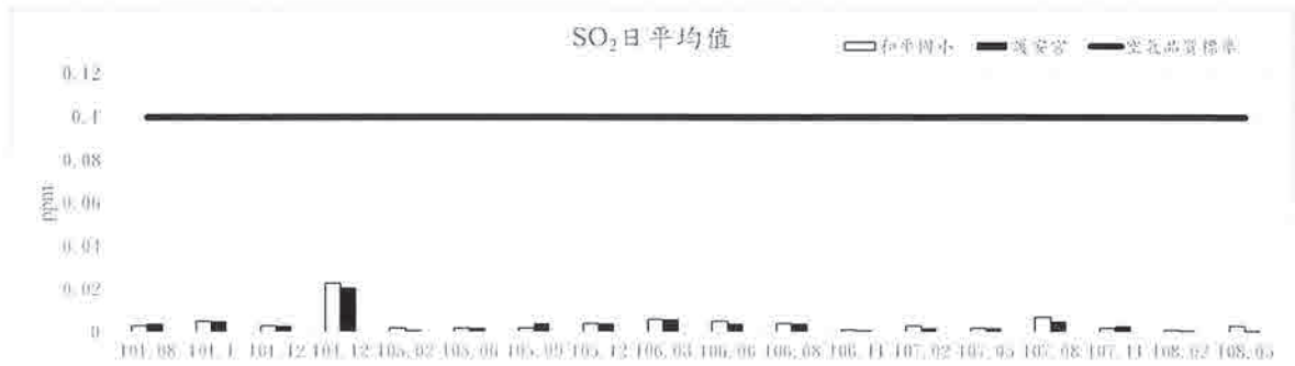
圖2.1-4 和平國小及護安宮之SO 2 平均值監測結果
