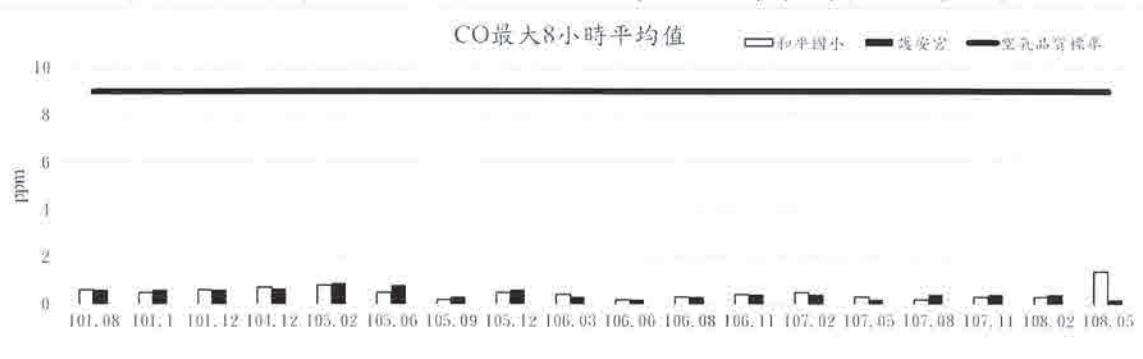
圖2.1-7 和平國小及護安宮之CO 8小時平均值監測結果
