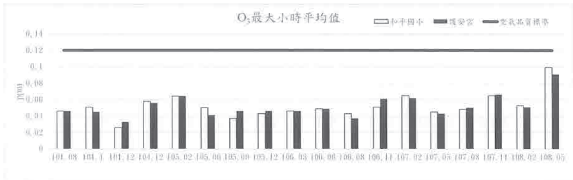
圖2.1-8 和平國小及護安宮之O 3 最大小時平均值監測結果
