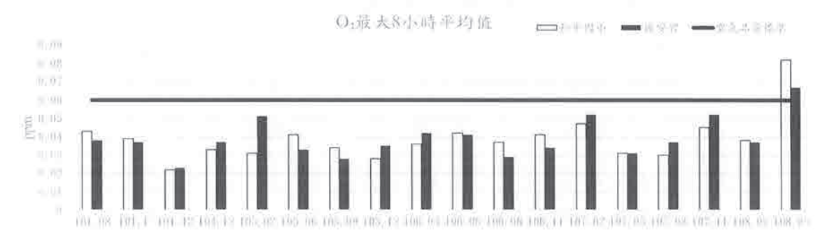
圖2.1-9 和平國小及護安宮之O 3 8小時平均值監測結果
