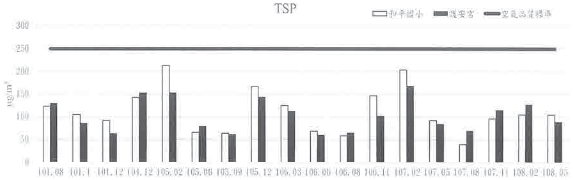
圖 2.1-1 和平國小及護安宮之 TSP 監測結果
