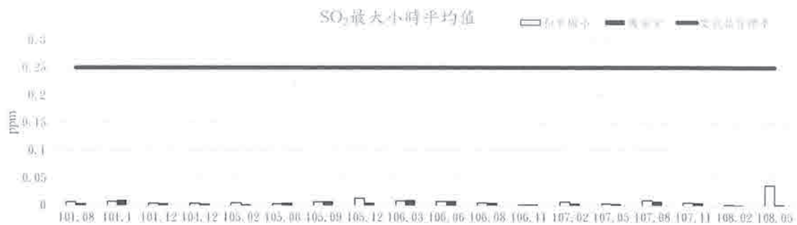
圖2.1-3 和平國小及護安宮之SO 2 最大小時平均值監測結果
