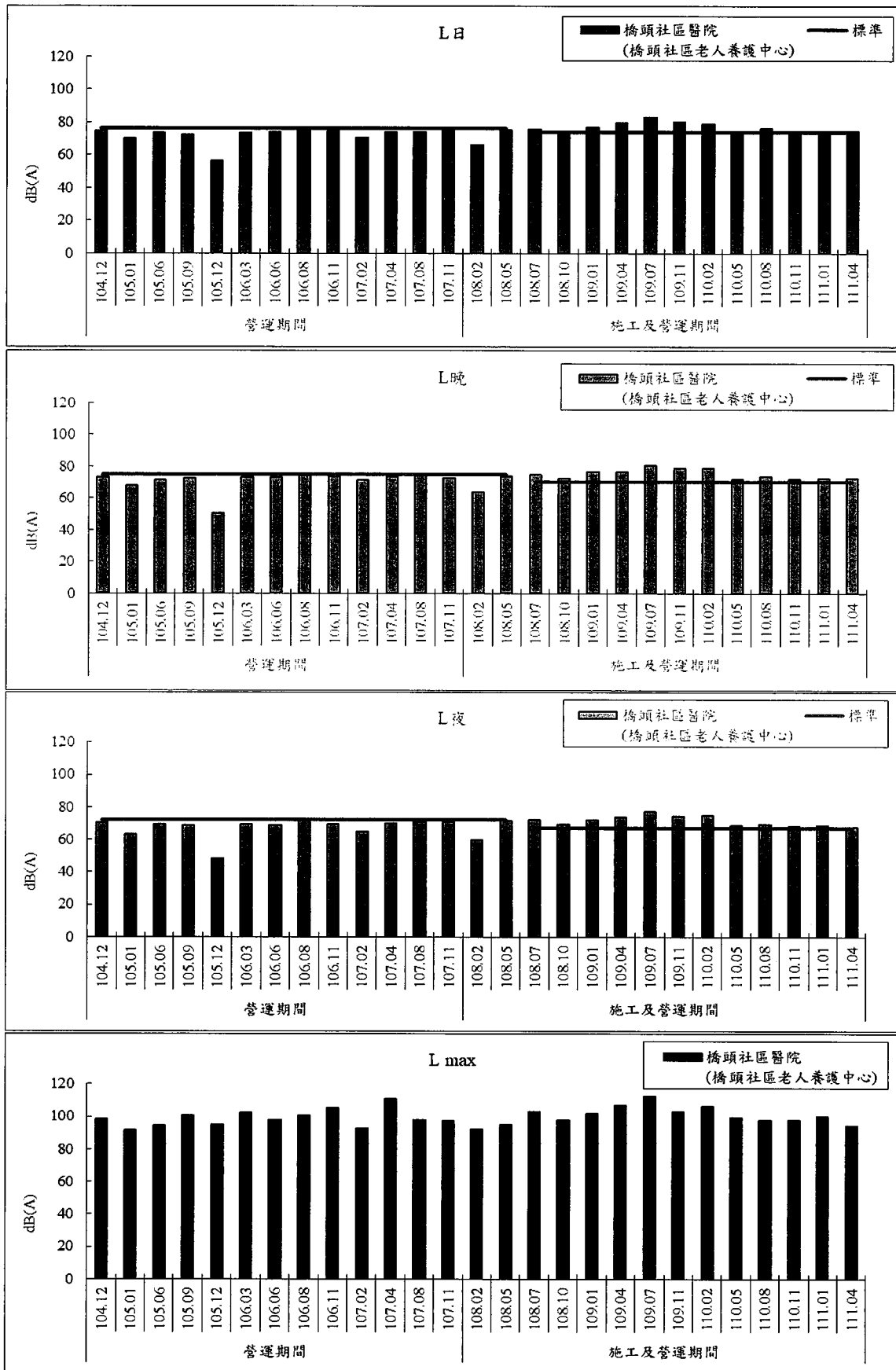
圖2.2-2 橋頭社區醫院(橋頭社區老人養護中心)噪音監測結果
