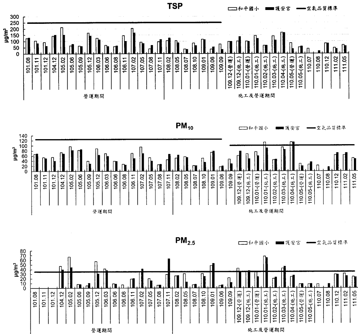
圖2.1-1 和平國小及護安宮之粒狀污染物監測結果
