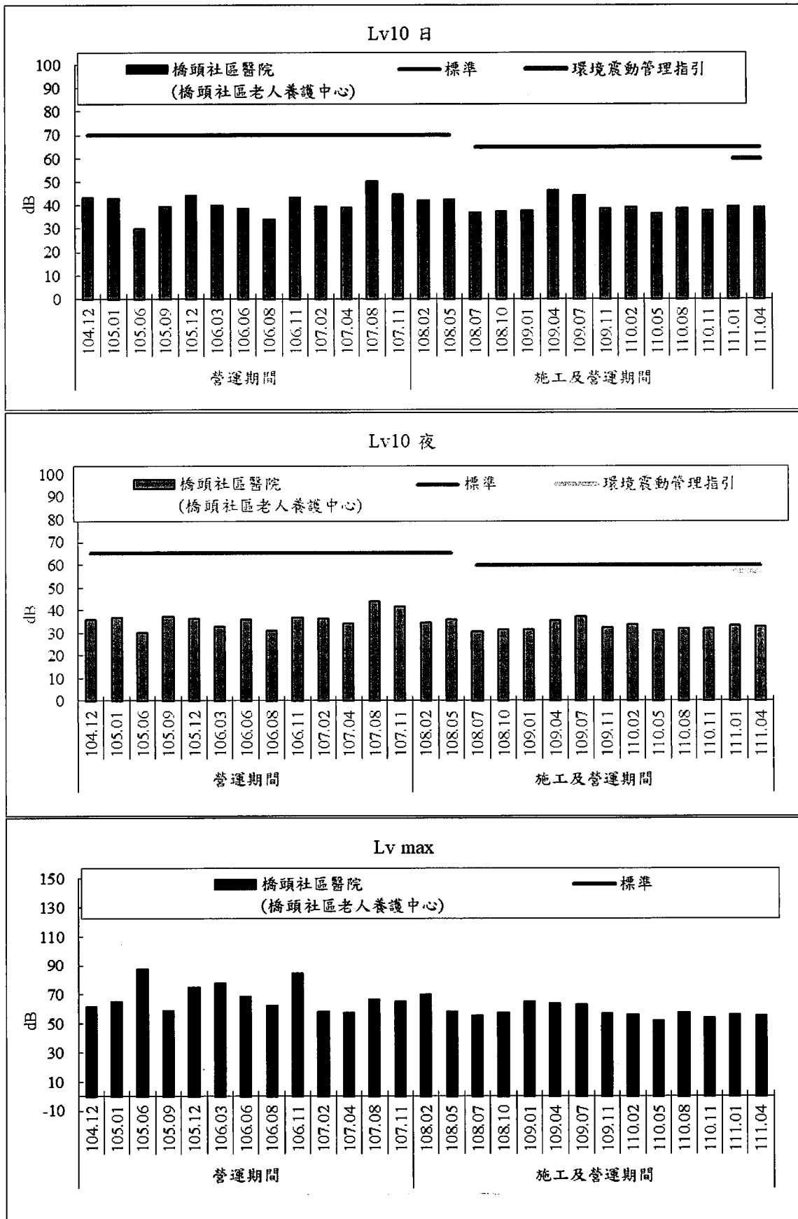
圖2.2-4 橋頭社區醫院(橋頭社區老人養護中心)振動監測結果
