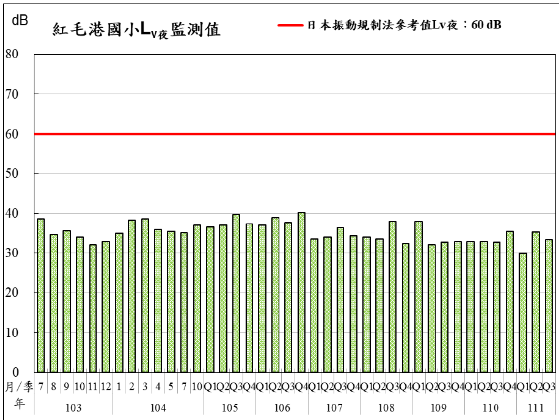
圖 2.2.2-1 紅毛港國小之歷次振動監測值變化
