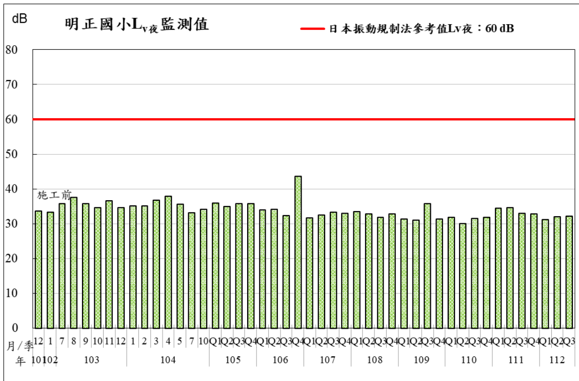
圖 2.2.2-2 明正國小之歷次振動監測值變化
