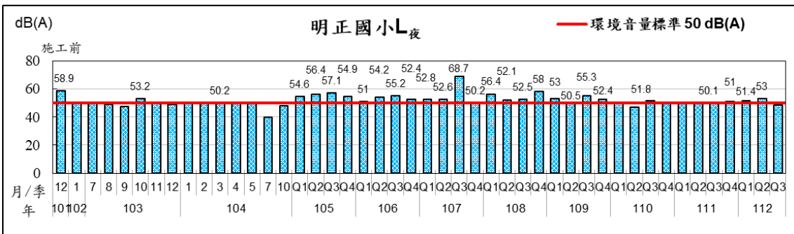
圖 2.2.1-2 明正國小之歷次噪音監測值變化
