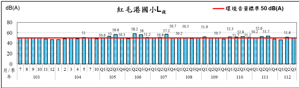
圖 2.2.1-1 紅毛港國小之歷次噪音監測值變化
